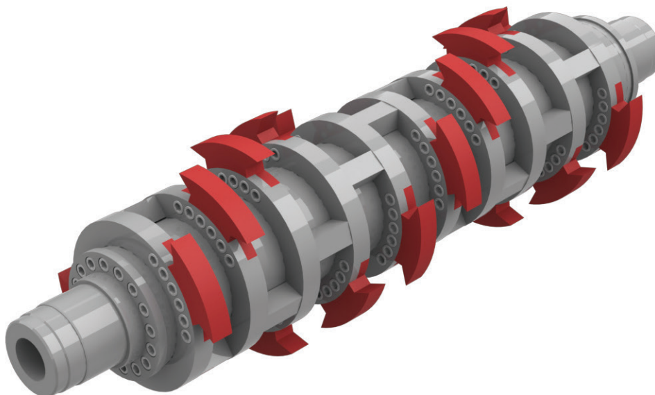
Валы шредера.
