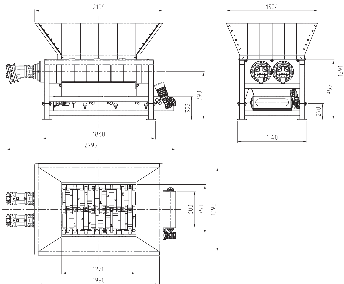
Габаритные размер shreddera.
